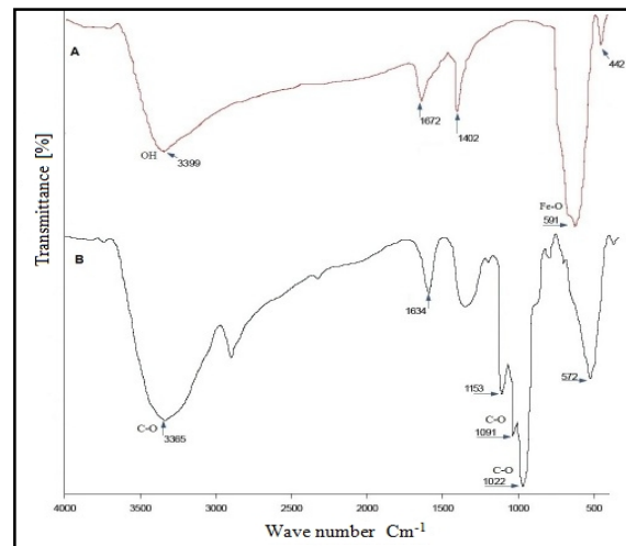
شکل ۲: طیف FT-IR از نانوذرات تهیه شده، الف) \text{Fe}_3\text{O}_4 بدون پوشش و ب) با پوشش نشاسته.
