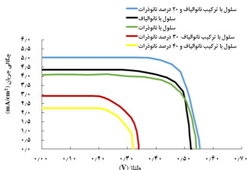
شکل ۱۰: نمودار جریان-ولتاژ پنج نمونه سلول ساخته شده با نانوذرات، نانوالیاف و ترکیب نانوالیاف و نانوذرات.
